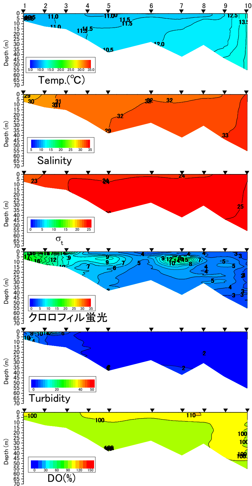
有明海中央ラインの水温(°C)、塩分、密度( \sigma_t )、クロロフィル蛍光強度、濁度、溶存酸素飽和度(DO%)の鉛直面図(国土交通省の調査による) (2017年2月27日)
